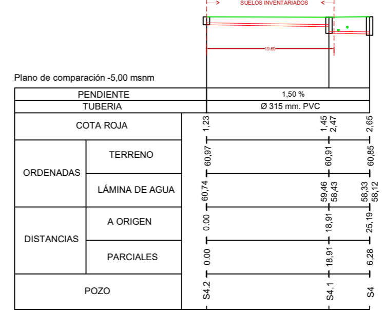
PERFIL LONGITUDINAL - SANEAMIENTO S4
