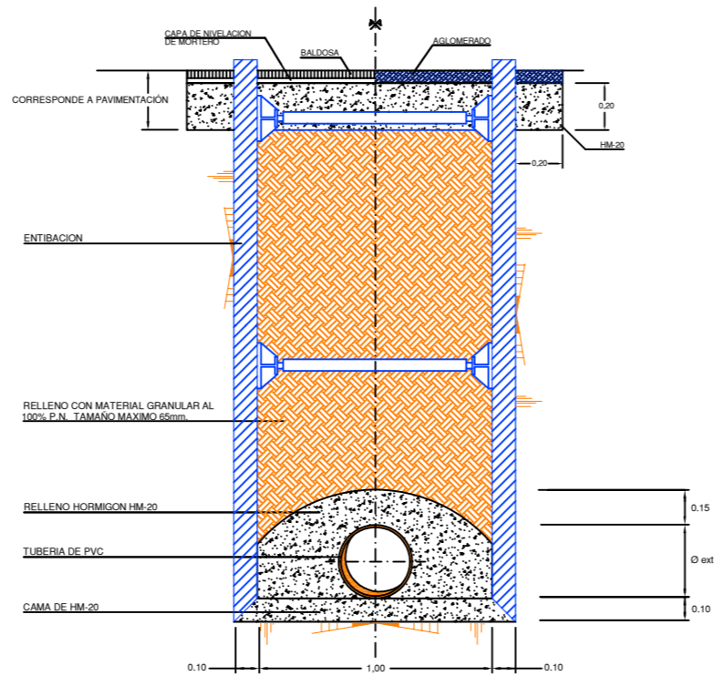
SECCION ZANJA TIPO SANEAMIENTO VII 2,00 < H < 3,00 m.
