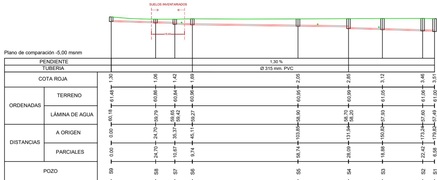
PERFIL LONGITUDINAL - SANEAMIENTO S1 - S9
