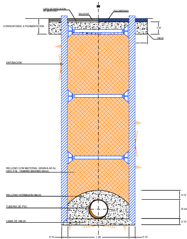
SECCION ZANJA TIPO SANEAMIENTO VIII 3,00 < H < 4,00 m.
