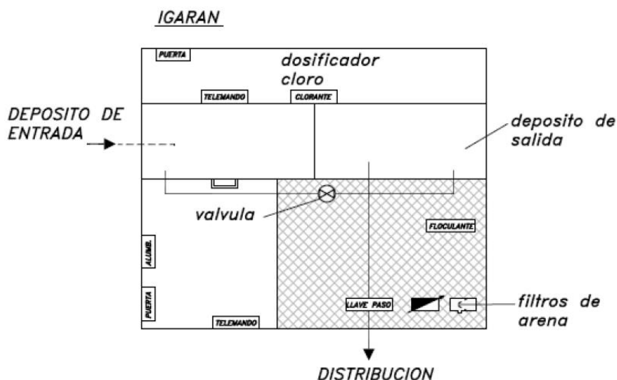
Ilustración 5. Distribución del depósito Igaran
