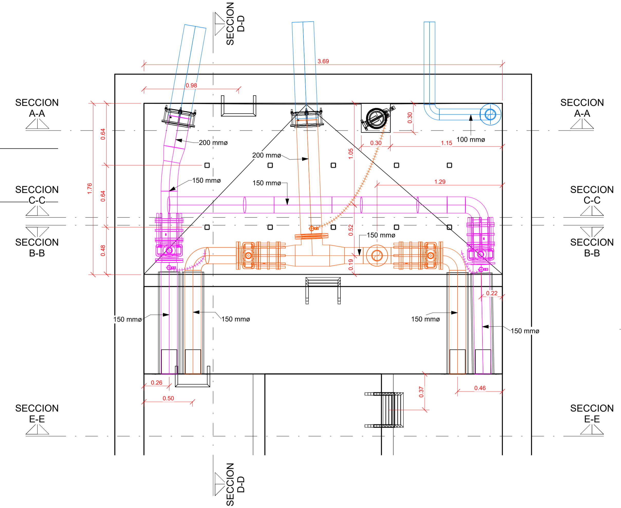
PLANTA CAMARA DE LLAVES 1:20
