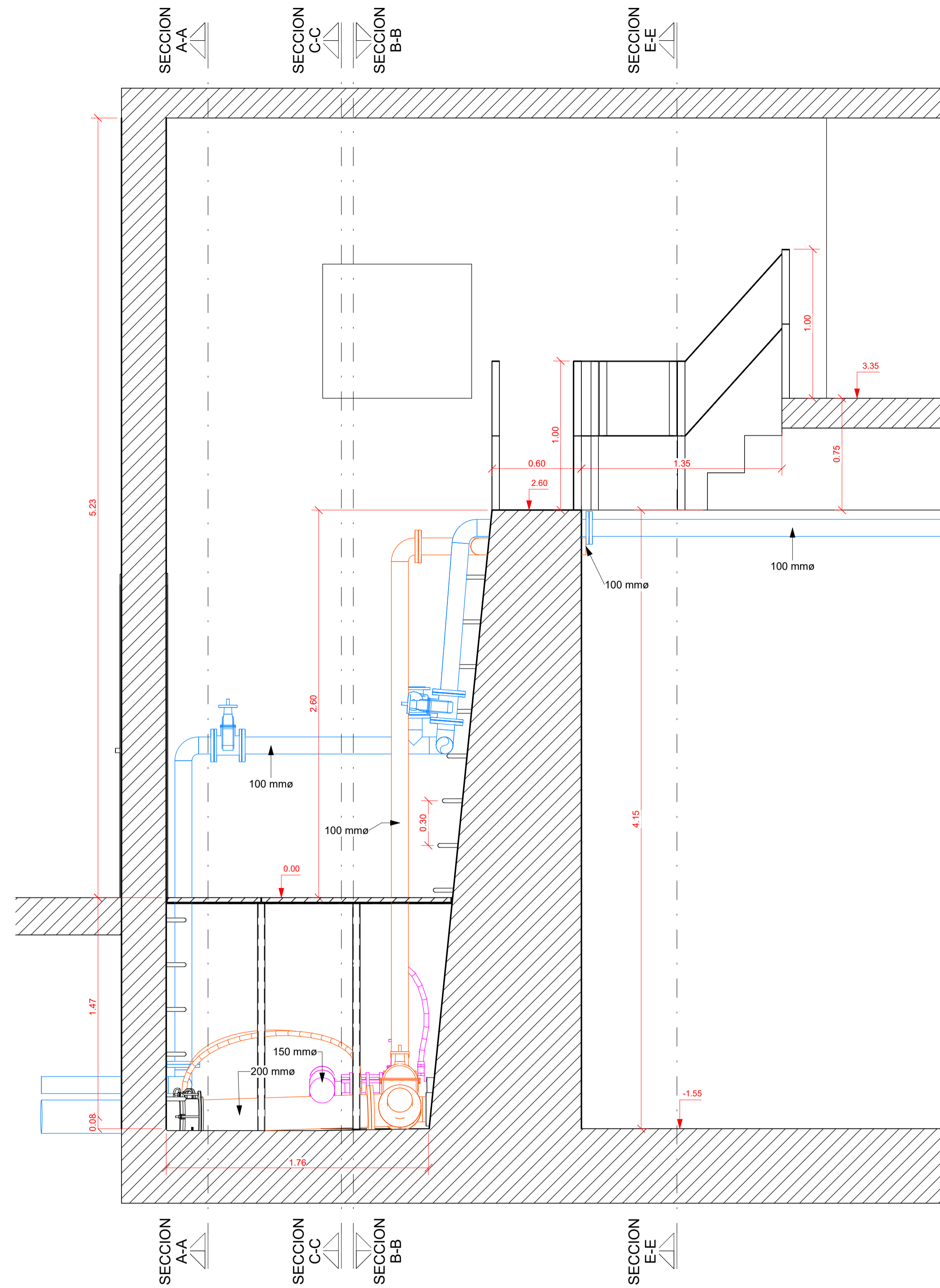
SECCION D-D 1:20
