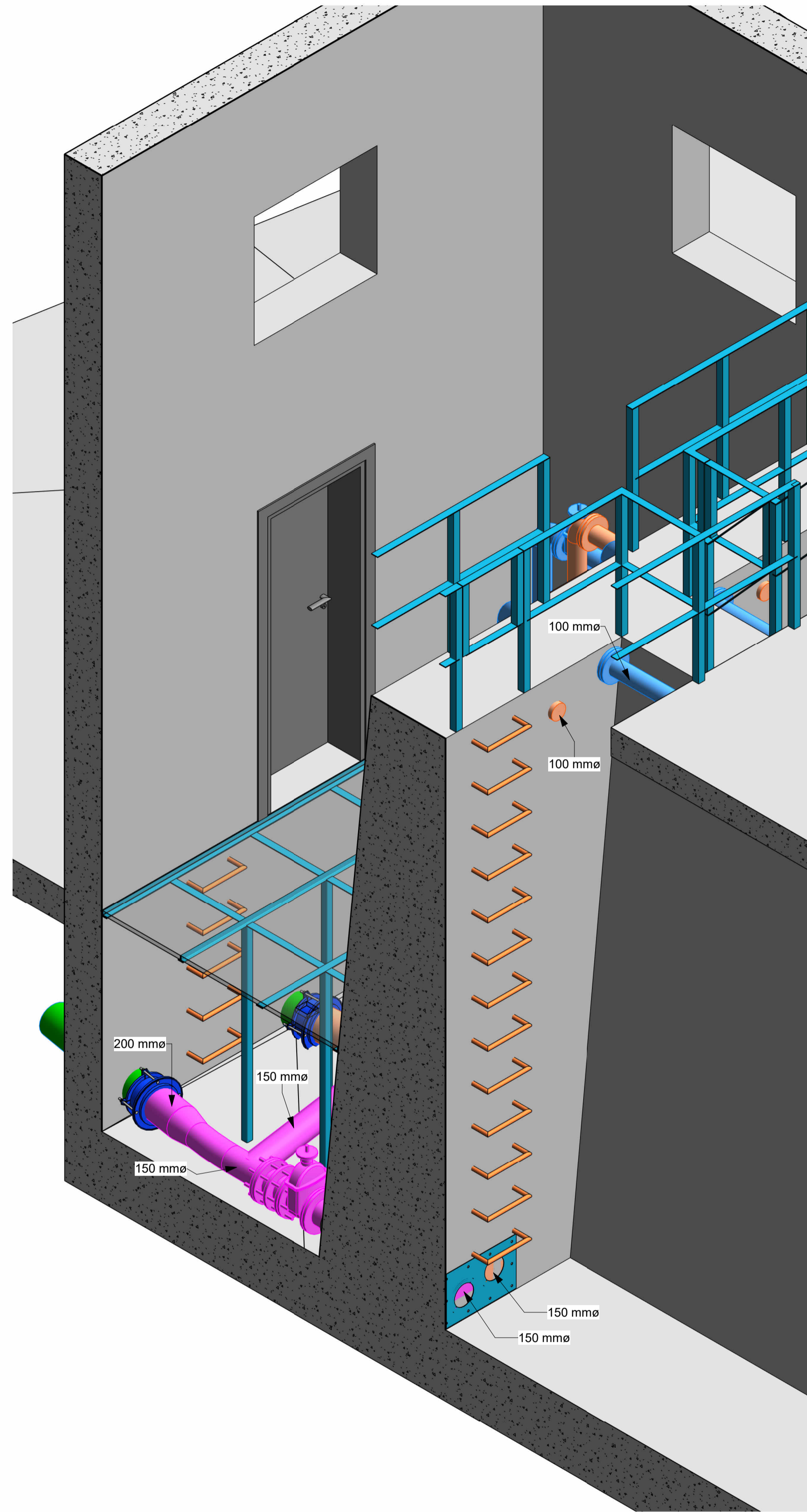
PERSPECTIVA 2
