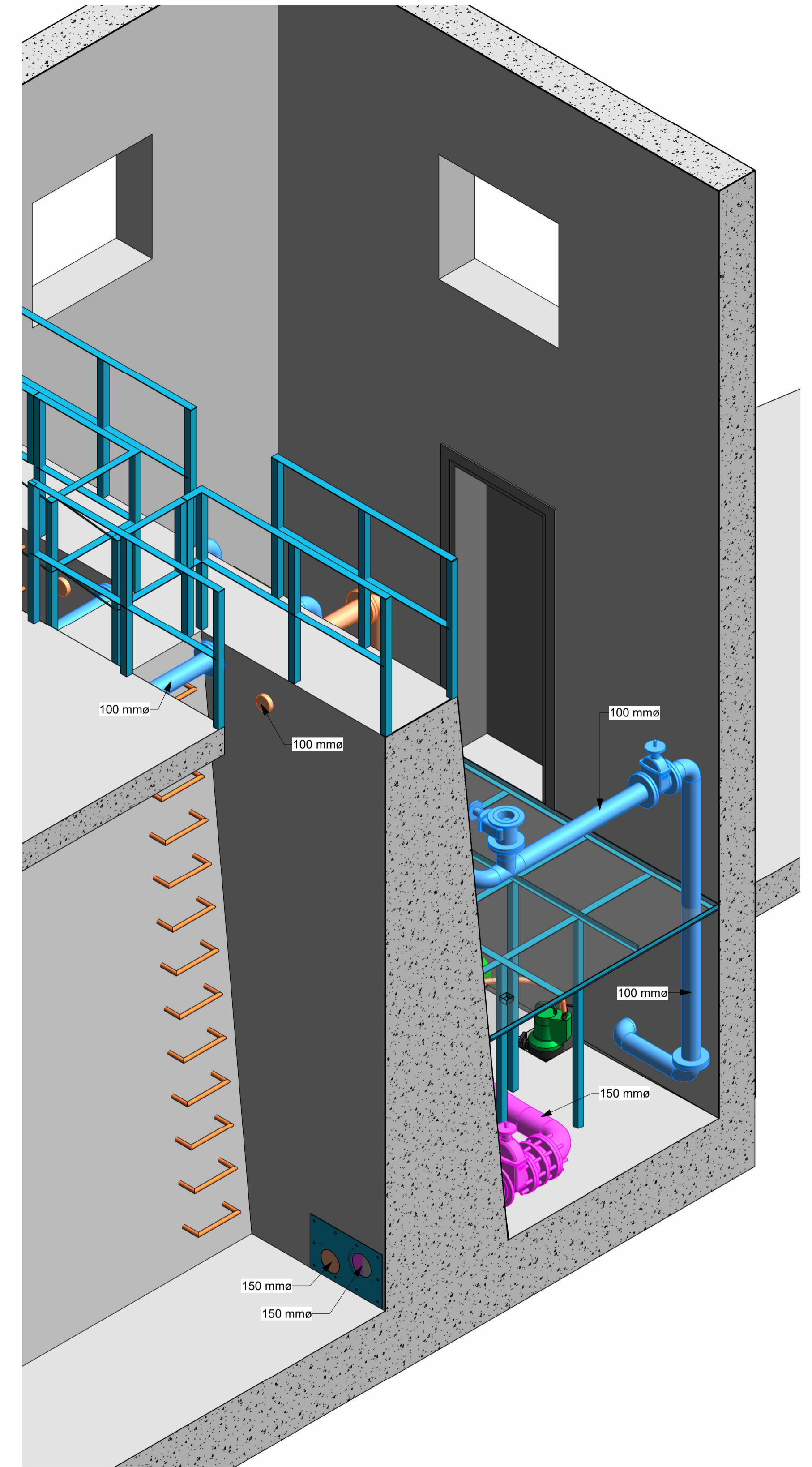
PERSPECTIVA 3
