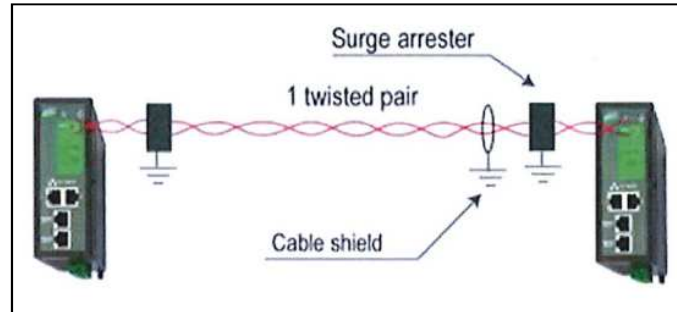
Ilustración 1. Conexión de protección contra sobretensiones.
